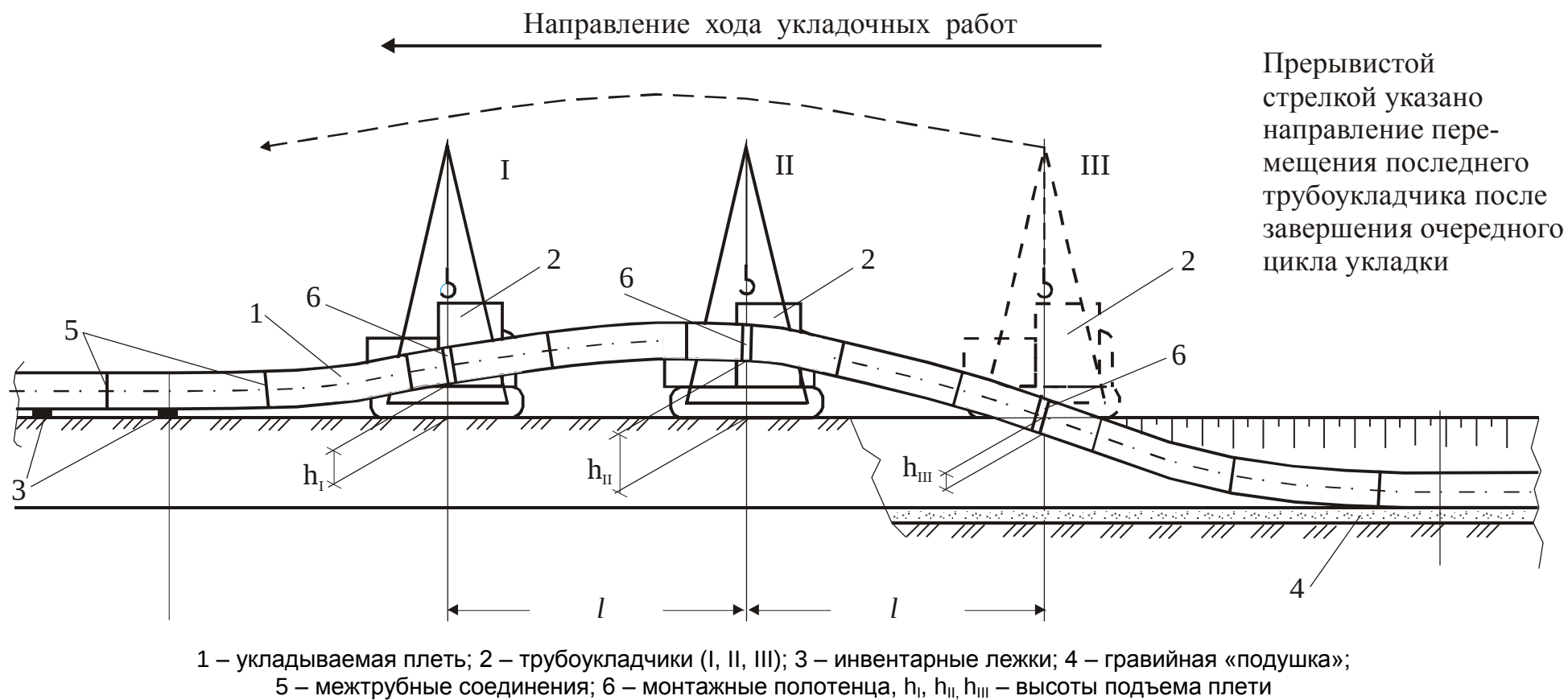
Рисунок 8 - Технологическая схема укладки длинномерных плетей при строительстве трубопроводов из стеклопластиковых труб
