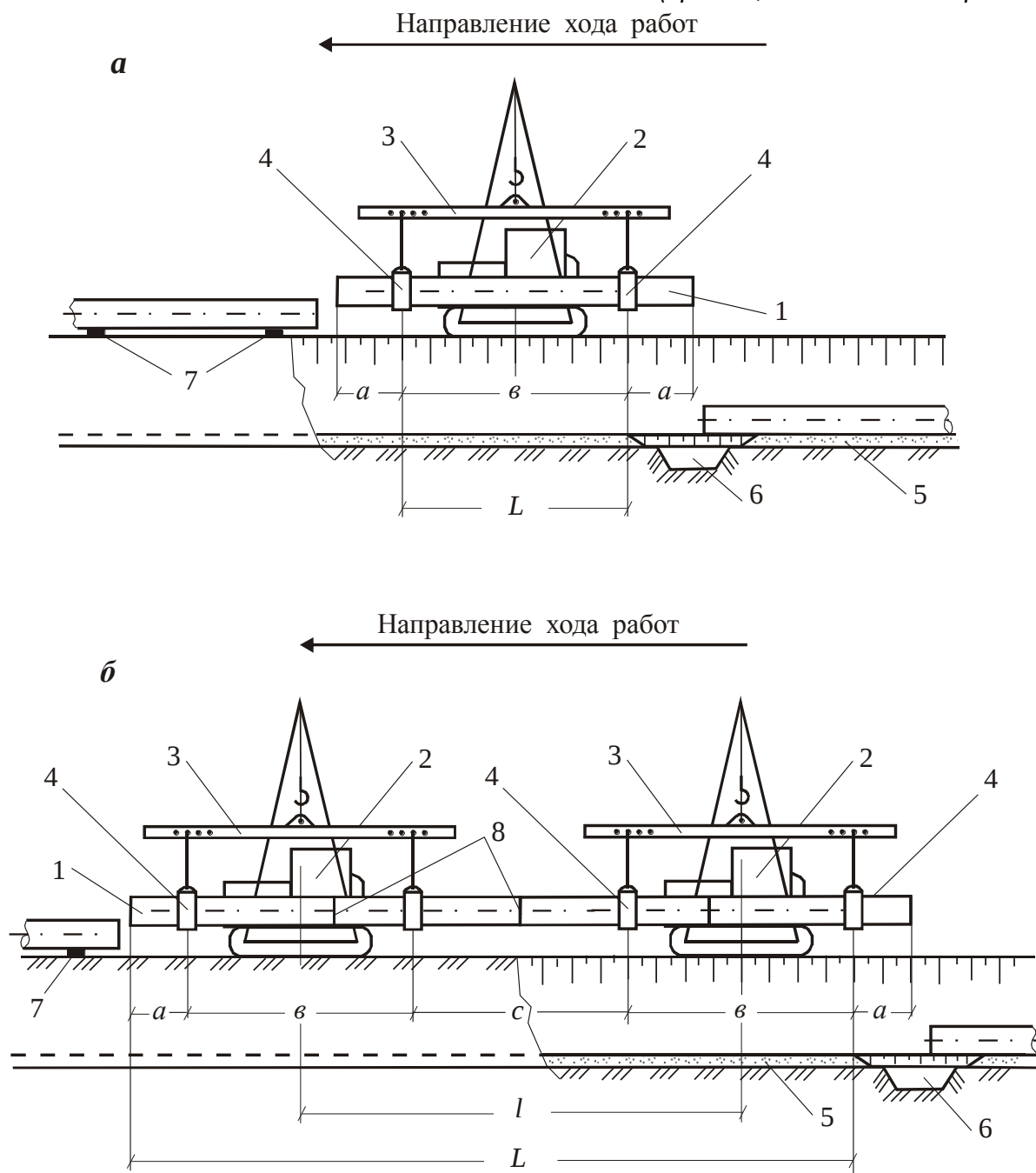
а) – при укладке одиночных труб; б) – при укладке секций 1 – укладываемая труба (секция); 2 – трубоукладчики; 3 – траверса; 4 – монтажное полотно; 5 – гравийная «подушка»; 6 – прямок; 7 – лежка; 8 – межтрубные соединения
