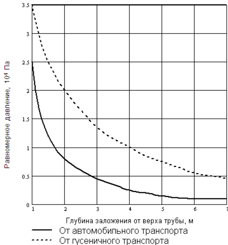
Рисунок 5 - Зависимость нормативного равномерно-распределенного давления транспорта от глубины заложения трубопровода
